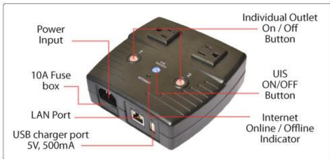
Fig.4 UIS-522B Hardware
