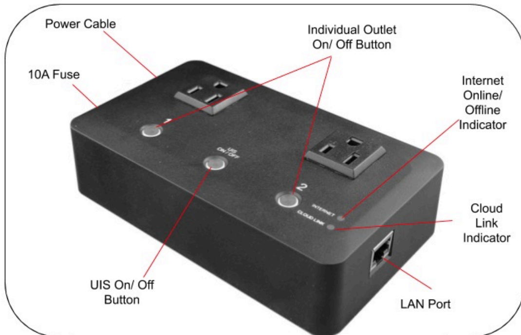
Fig.5 UIS-622B Hardware
